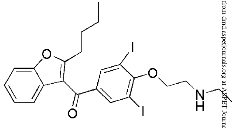
desethylamiodarone
