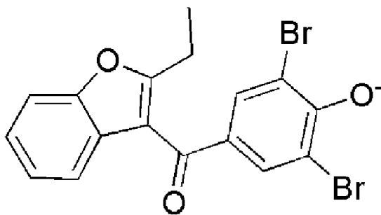
benzbromarone
