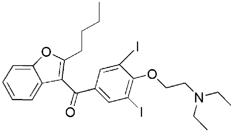
amiodarone
