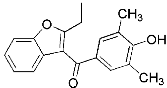
benz(meth)arone
