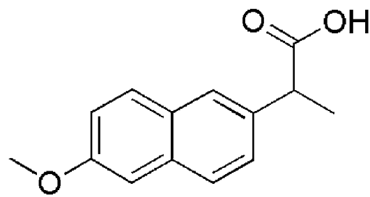
naproxen
