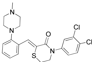
Elzasonan
