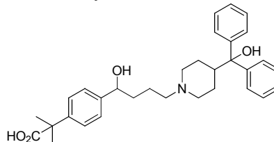
Fexofenadine
