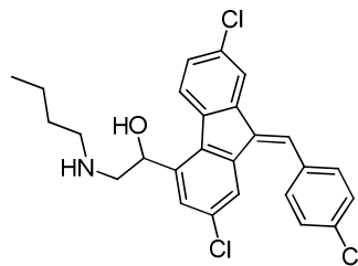
Desbutyllumefantrine
