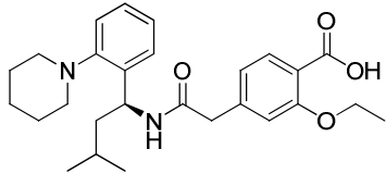
Regalinide
