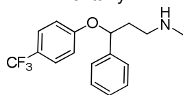
Fluoxetine
