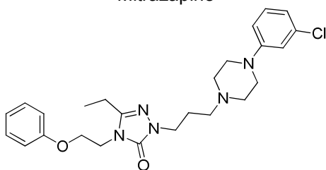
Nefazodone
