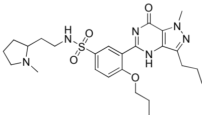
Udenafil
