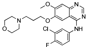
Gefitinib
