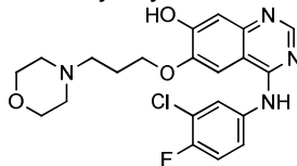
Demethoxygefitinib
