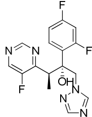
Voriconazole
