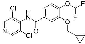
Roflumilast
