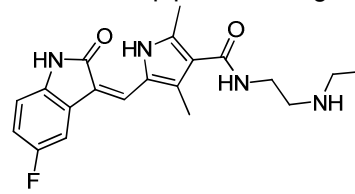
Desethylsunitinib
