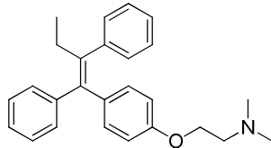
Tamoxifen
