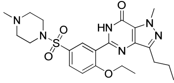
Sildenafil
