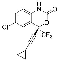
Efavirenz
