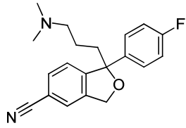
Citalopram
