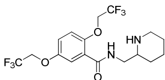
Flecainide
