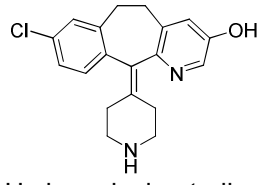
Hydroxydesloratadine
