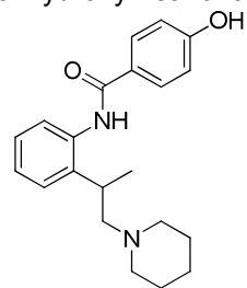
Demethyencanide
