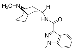
Granisetron
