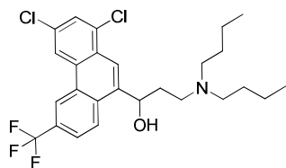
Halofantrine
