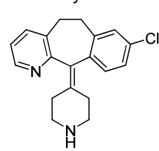
Desloratadine
