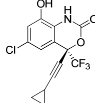
HydroxyEfavirenz
