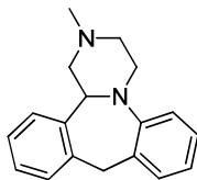
Mianserin
