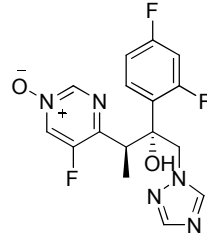
Voriconazole N-oxide
