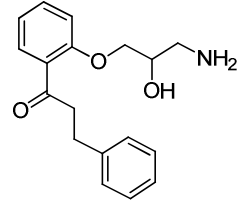
Despropylpropafenone
