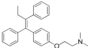
Tamoxifen
