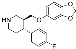
Paroxetine
