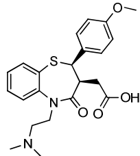
Diltiazem
