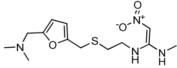
Ranitidine
