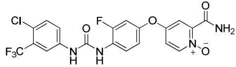
N-Desmethylregorafinib N-oxide
