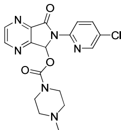
Zopiclone
