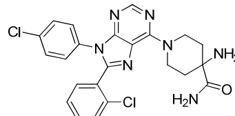
Desethylotenabant
