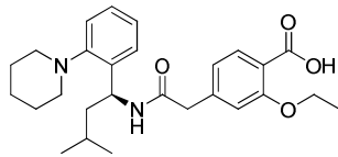
Regalinide
