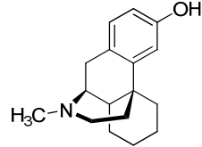
Demethoxydextromethorphan
