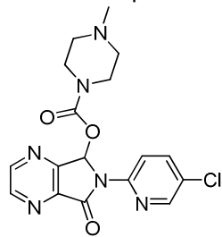
Zopiclone
