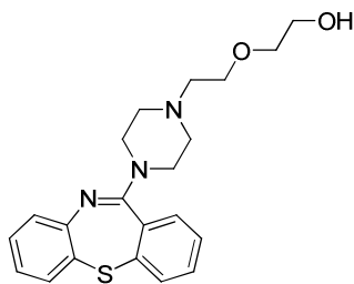
Quetiapine
