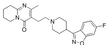
Risperidone
