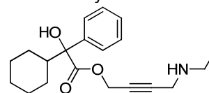
Desethyloxybutynin
