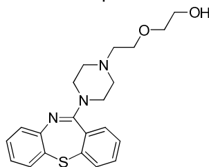
Quetiapine
