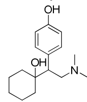
Desvenlafaxine
