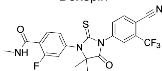
Enzalutamide
