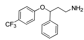
Norfluoxetine
