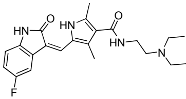
Sunitinib
