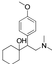
Venlafaxine
