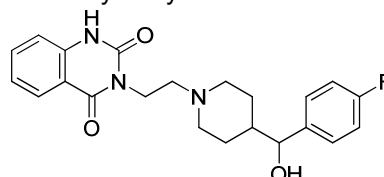
Ketanserinol
