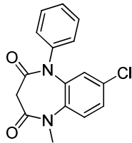
Clobazam
