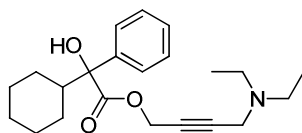
Oxybutynin
