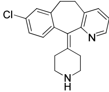
Desloratadine
