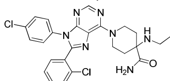
Otenabant (CP-945598)
