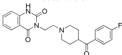
Ketanserine
