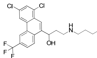
Desbutylhalofantrine
