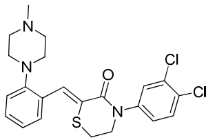
Elzasonan
