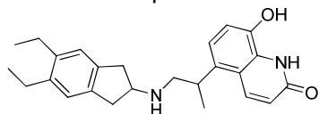
Indacaterol
