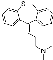
Dothiepin
