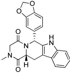
Tadalafil
