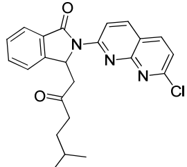
Pagoclone
