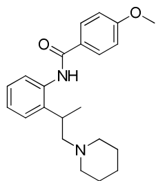
Encainide
