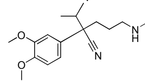
D617
