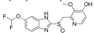
Demethoxypantoprazole
