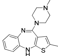
Olanzapine
