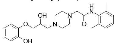
Demethoxyranolazine
