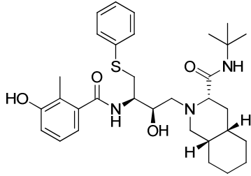
Nelfinavir
