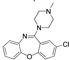
Loxapine
