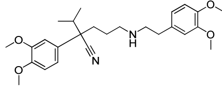
Norverapamil
